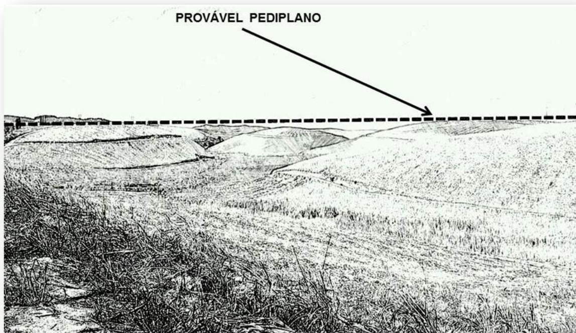
Figura 24. Provável pediplano em ambiente tropical úmido. Zona da Mata de Pernambuco.
