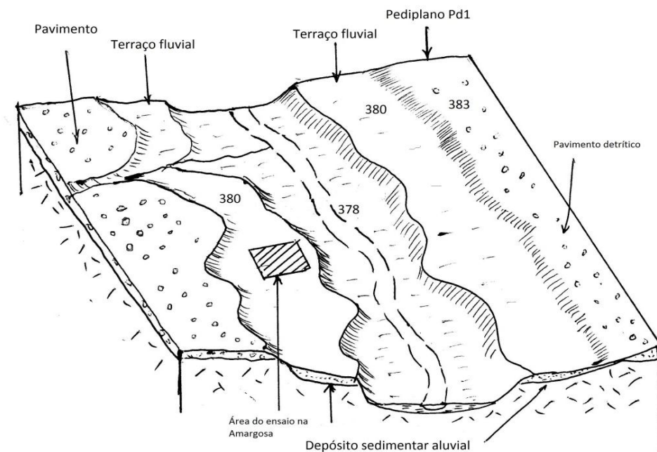
Figura 49. Bloco diagrama apresentando detalhe da compartimentação geomorfológica da área adjacente ao Riacho Pontal.
