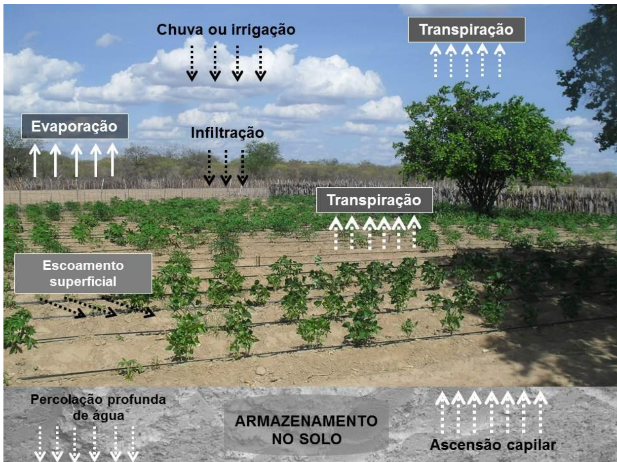
Figura 41. Dinâmica do movimento da água no sistema solo-planta-atmosfera, em paisagens naturais.
