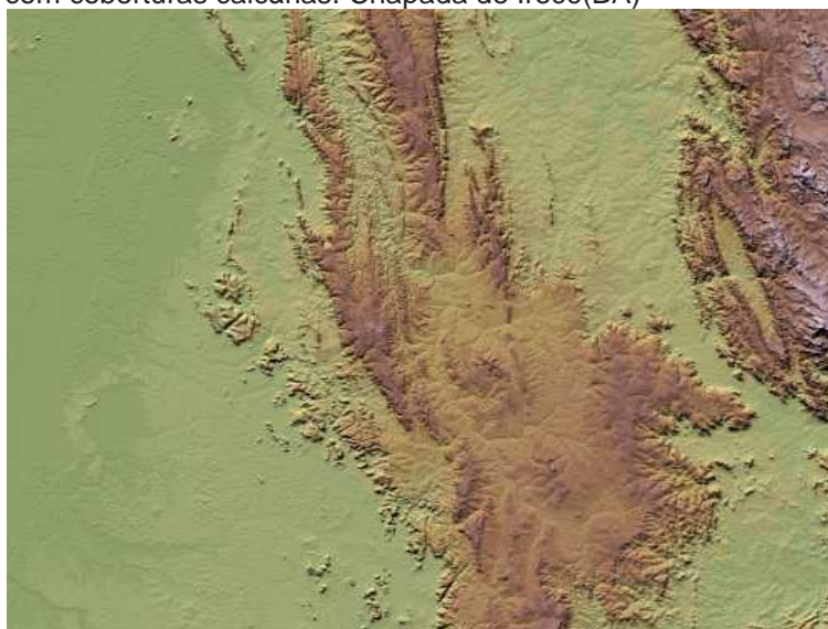
Figura 27. Planaltos com coberturas calcárias. Chapada de Irecê(BA)
