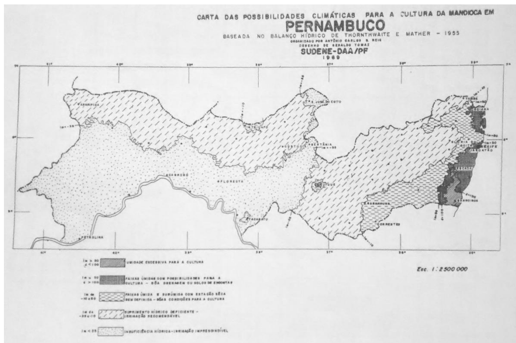
Figura 63. Possibilidades climáticas para a cultura da mandioca.
