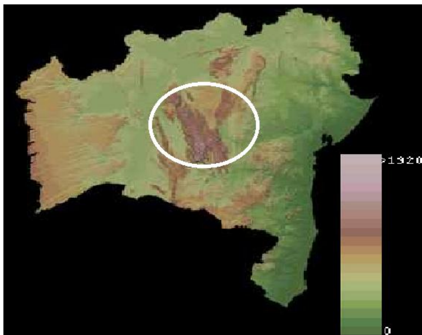
Figura 29. A unidade de paisagem Chapada Diamantina e adjacências
