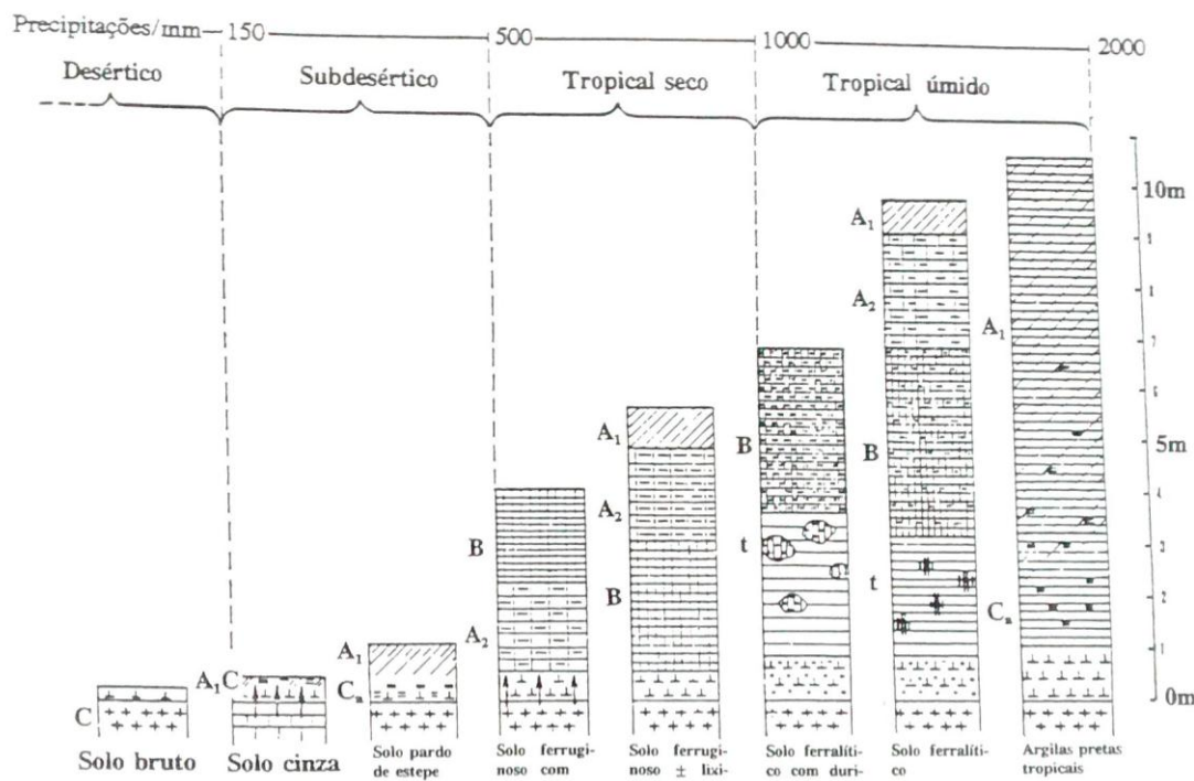
Fig. 9-16. Zonação geográfico-climática dos principais solos africanos entre as regiões áridas do Saara e as tropicais (segundo Lacoste & Salanon, 1973).
