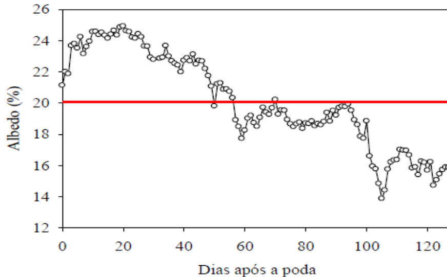
Figura 37. Valores médios diários de albedo da videira Syrah no Submédio Vale do São Francisco em função dos dias após a poda. Onde a linha vermelha indica o albedo médio diário durante o ciclo.
