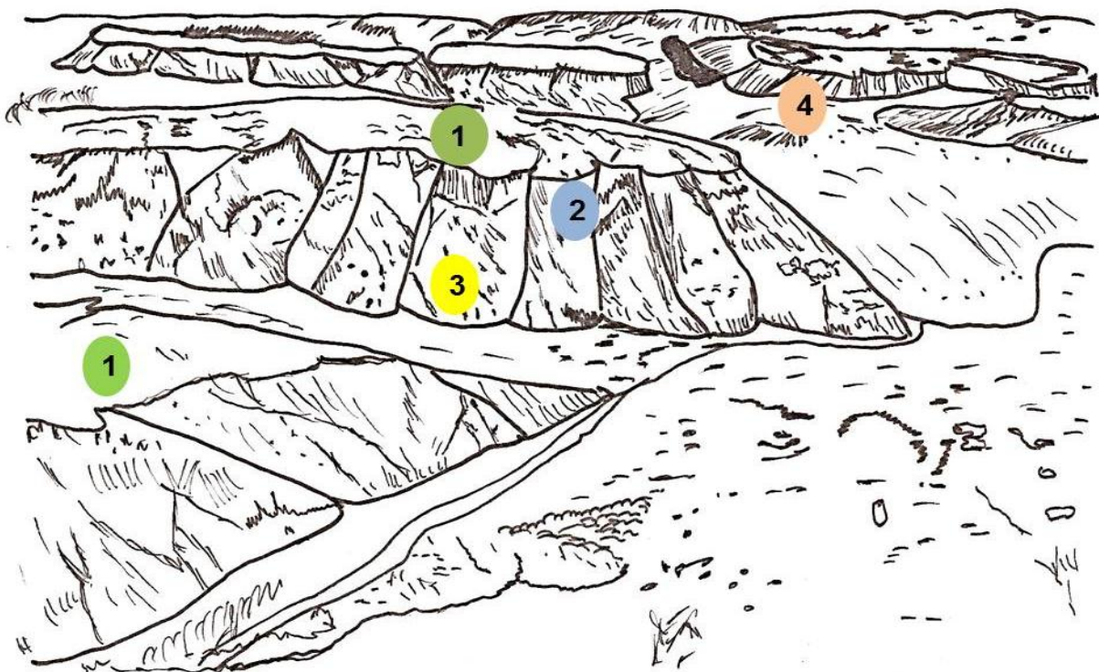
Figura 5. Retalhos da superfície de erosão no geossistema. Cristalino Setentrional, a oeste da cidade de Timbaúba (PE). Ilustração: Lucivânio Jatobá (2017)
