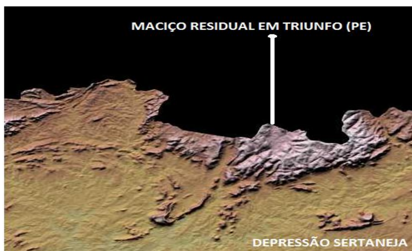
Figura 28. Maciço Residual. Triunfo(PE)
