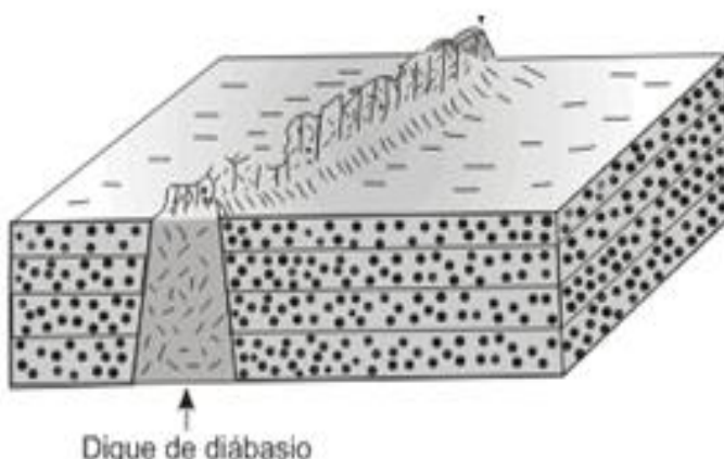
Figura 14. Crista desenvolvida em dique de diabásio
