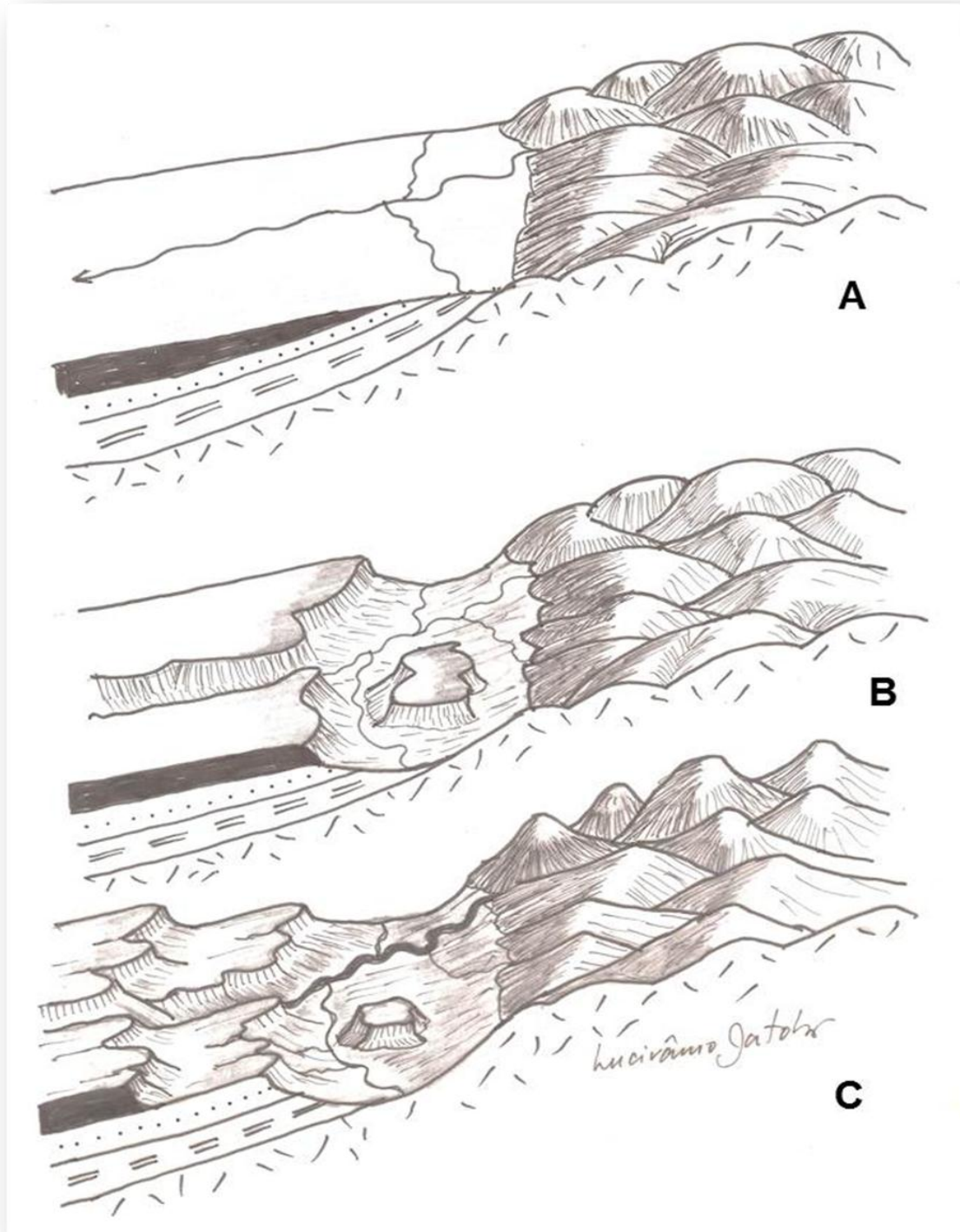
Figura 19. Gênese e evolução de paisagens cuestiformes
